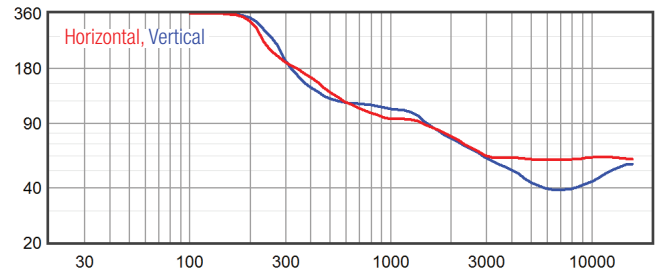
Beamwidth
