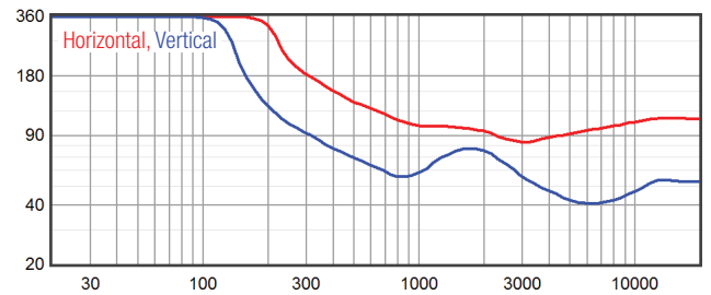
Beamwidth
